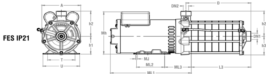
IMAGEM 1 – DIMENSÕES DA MOTOBOMBA
