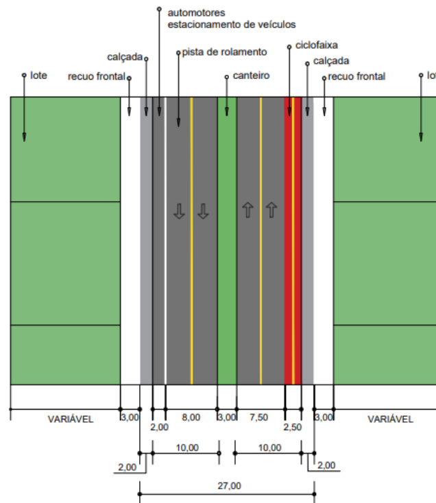
Detalhe Avenida dos Imigrantes
