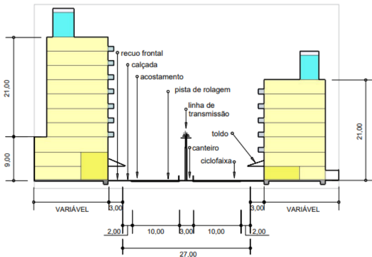
Perfil básico da Avenida dos Imigrantes
