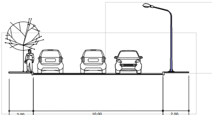
Perfil básico das ruas arteriais, coletoras e locais
