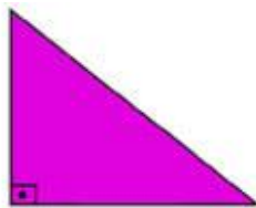
Retângulo
