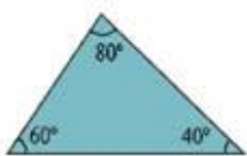
Acutângulo
