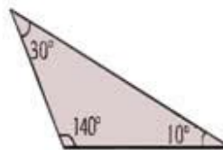
Obtusângulo
