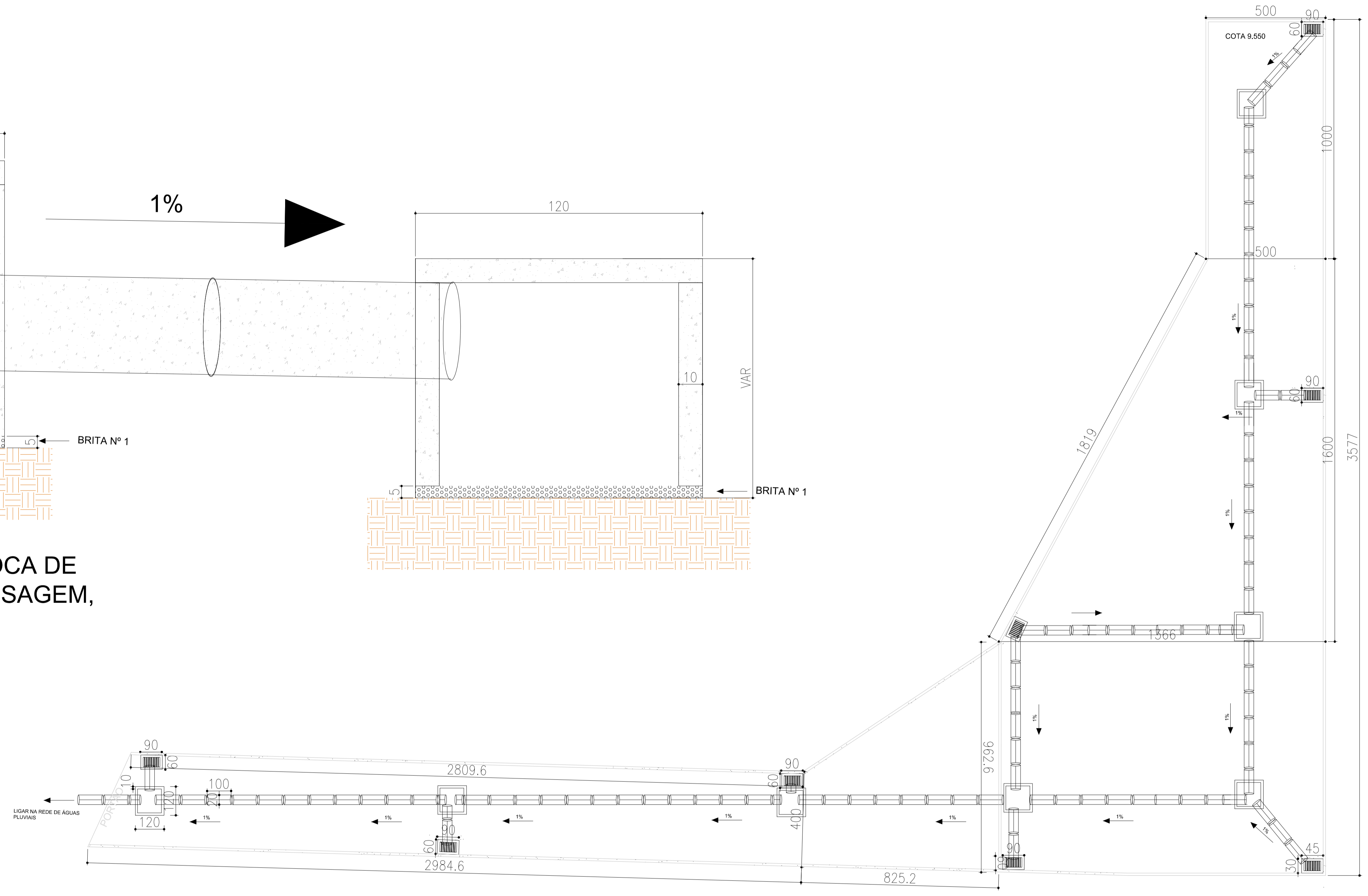
IMPLANTAÇÃO DA REDE DE DRENAGEM NO ACESSO, ESC. 1/100
