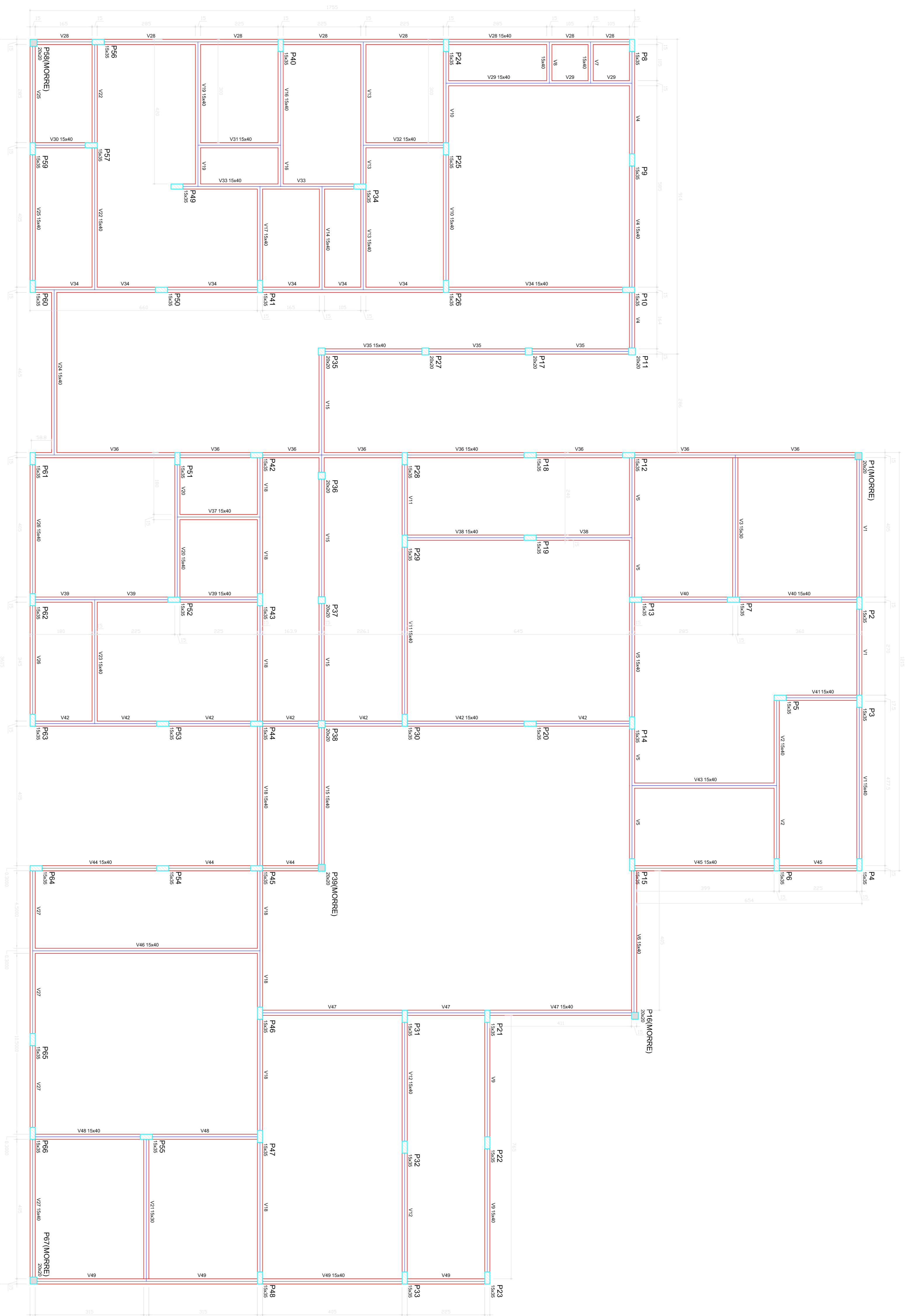
Forma do pavimento Baldrame escala 1:75
